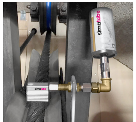
Das Seil einer Standseilbahn wird durch einen simalube Schmierstoffgeber geschmiert. Mit der Bürste wird der Schmierstoff aufgetragen und das Seil gereinigt.
