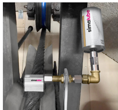
Le câble d'un téléphérique est lubrifié avec un graisseur simalube. La brosse sert à appliquer la graisse et à nettoyer le câble.
